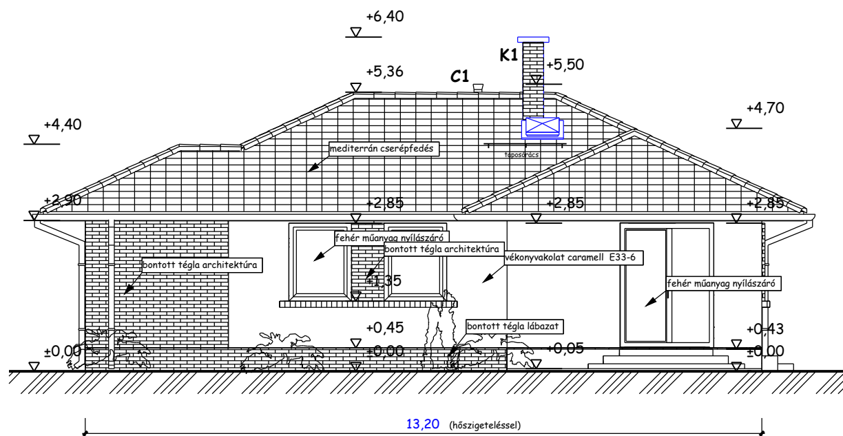
Tervezett délkeleti homlokzat
