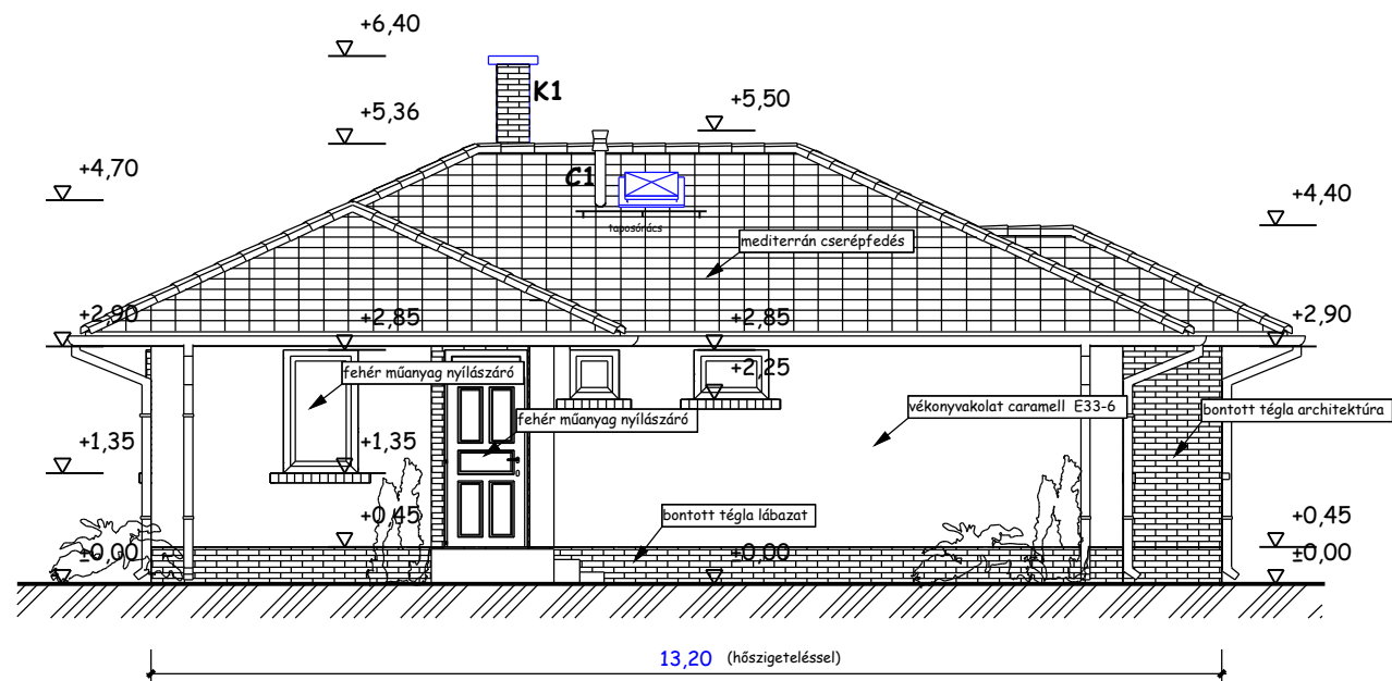
Tervezett északnyugati homlokzat
