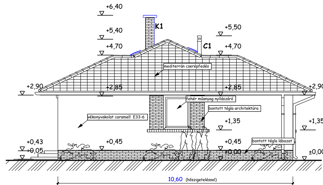
Tervezett északkeleti homlokzat
