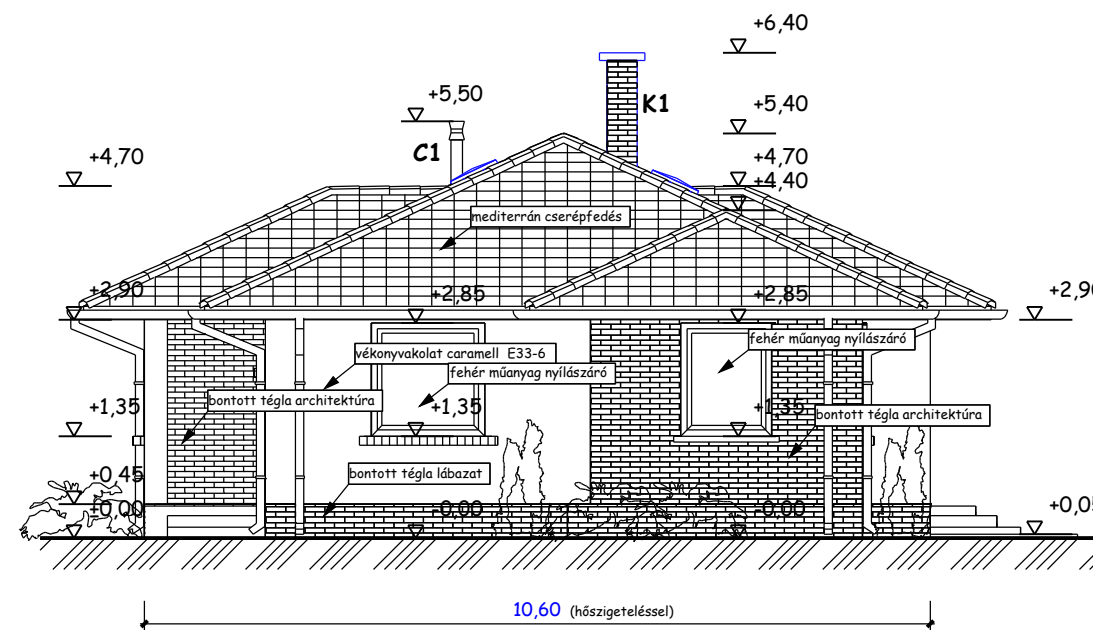
Tervezett délnyugati homlokzat
